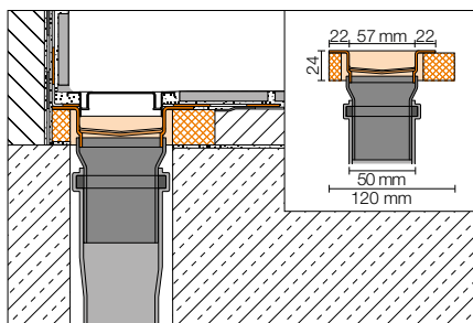
Példa: KERDI-LINE-VS
