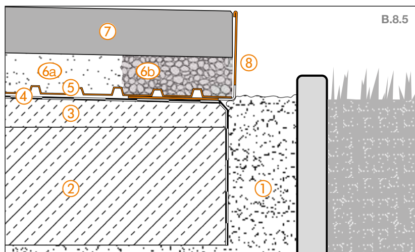
Detal krawędzi 4
