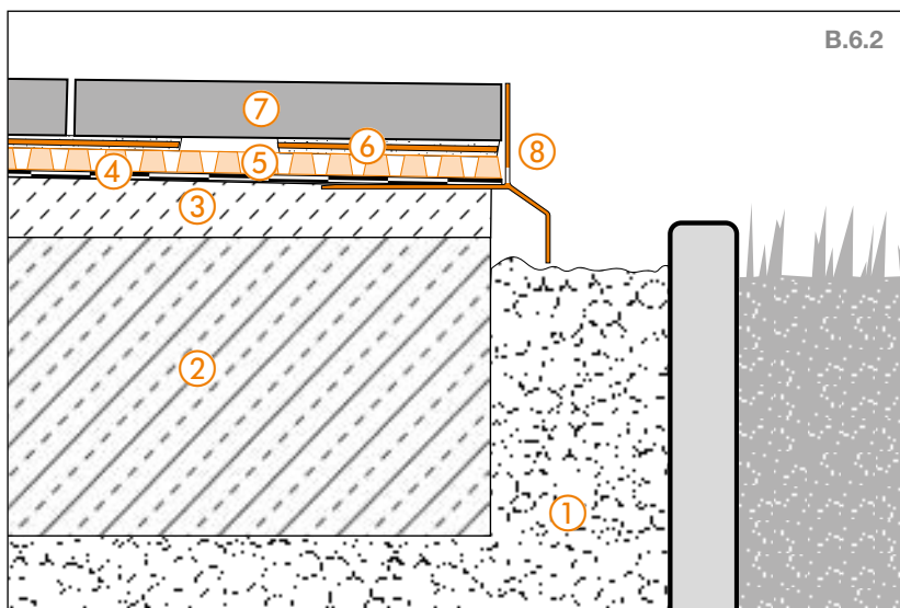
Detal krawędzi 1
