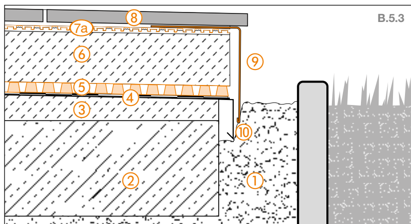
Detal krawędzi 2
