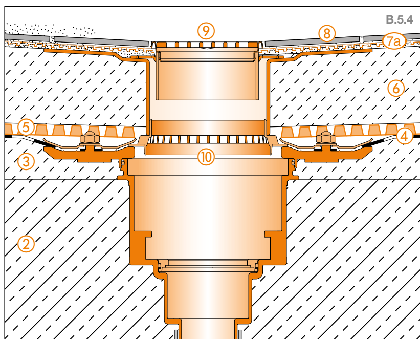
Wpust podłogowy
