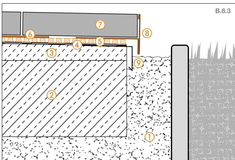
Detal krawędzi 2
