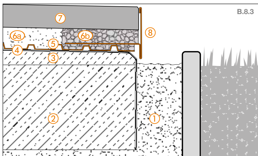
Detal krawędzi 3
