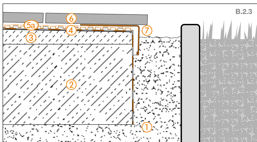
Detal krawędzi 2
