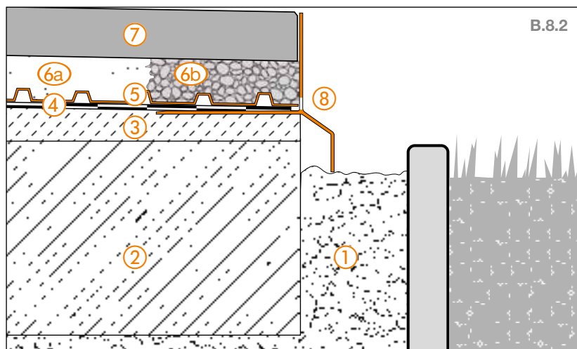
Detal krawędzi 1
