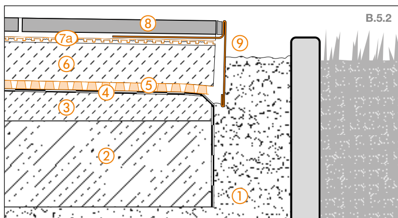
Detal krawędzi 1
