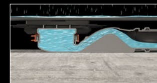
Efecto autolimpieza a través de la alta velocidad de flujo del agua en el interior del bote de salida
