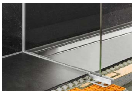
Schlüter-DECO-SG : Montage dans la zone de douche avec un élément en verre
