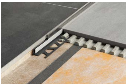
Schlüter-SHOWERPROFILE-S Inbouw in een gelijkvloerse douchevloer
