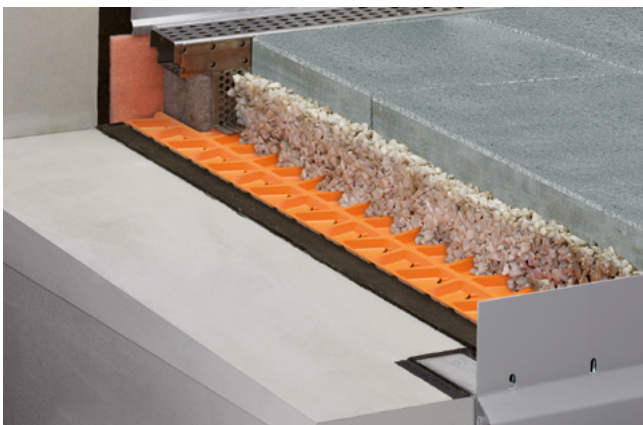
Bekledingsconstructie op kiesel-/splitbed met Schlüter-TROBA
