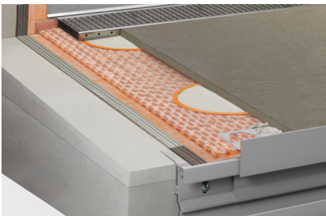
Losse plaatsing op Schlüter-KERDI en Schlüter-TROBA-PLUS 8G
