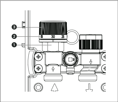
Fig. 3: Håndhjul
