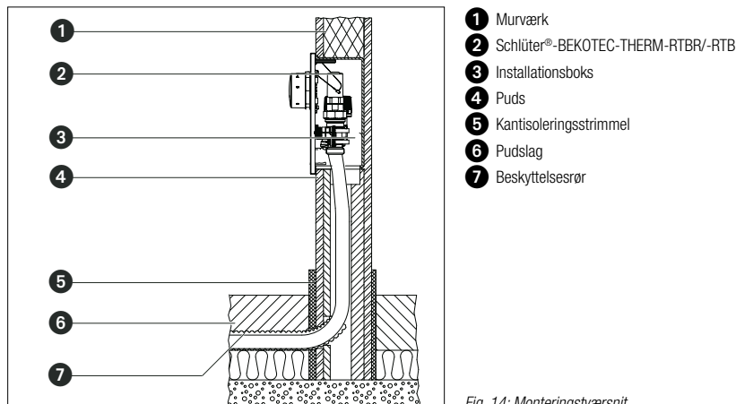
Fig. 14: Monteringstværsnit
