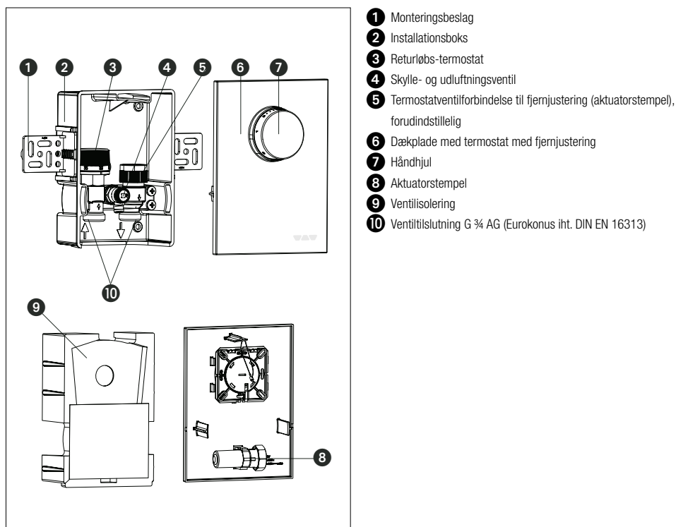
Fig. 1: Struktur BEKOTEC-THERM-RTBR
