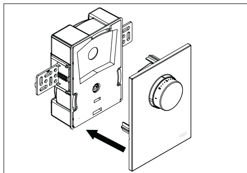
Fig. 20: Montering af dækplade med håndhjul
