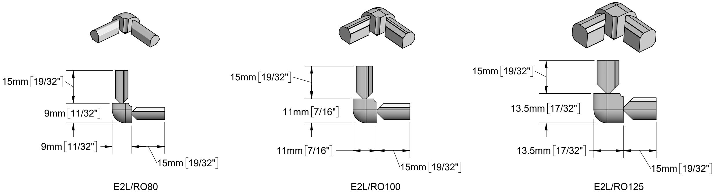
E2L/RO = DOUBLE-LEG OUTSIDE CORNERS, 90° / COINS EXTERNES À DEUX EMBOUTS, 90°
