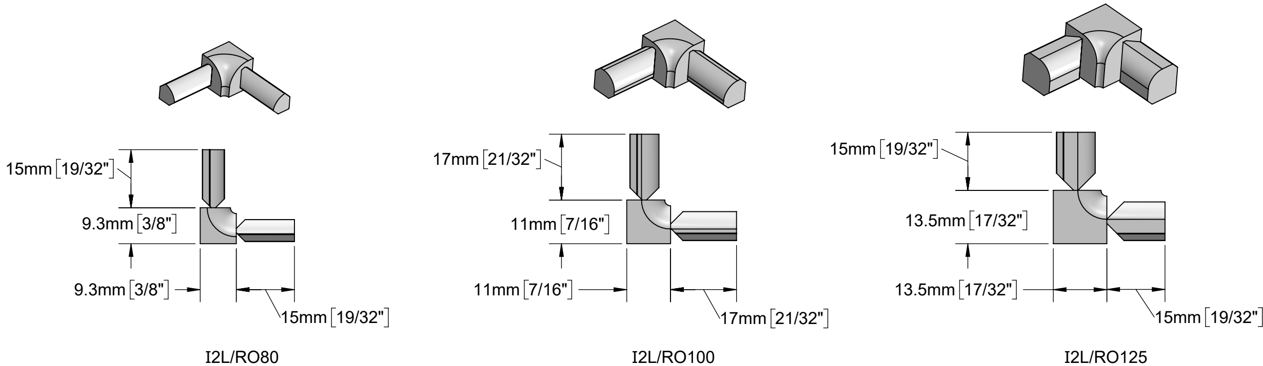
I2L/RO = DOUBLE-LEG INSIDE CORNERS, 90° / COINS INTERNES À DEUX EMBOUTS, 90°
