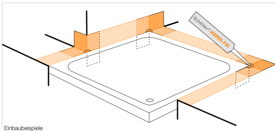
Einbaubeispiele
