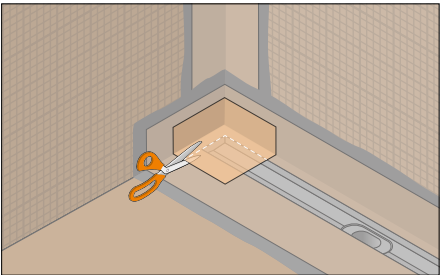
2 KERDI Manschette mit KERDI-COLL-L dicht verkleben. Die im Lieferumfang enthaltene Schlüter-KERDI-KERECK Innenecke zuschneiden ...
