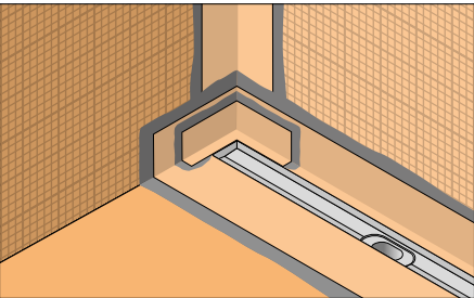
3 ... und mit KERDI-COLL-L aufkleben.
