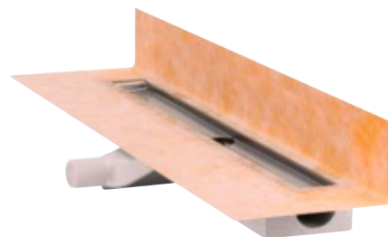
Schlüter-KERDI-Manschette, aufgestellt für Wandebau
