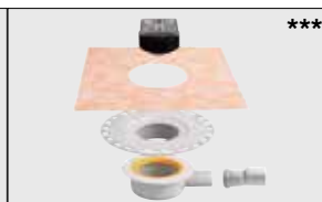
KERDI-DRAIN-BASE 1 sada (s design mřížkou 1)
