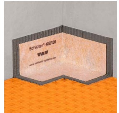
Schlüter®-KERDI-KERECK/FI (2 pcs.)
