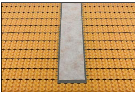
Pontage des raccords avec Schlüter®-KERDI-KEBA
