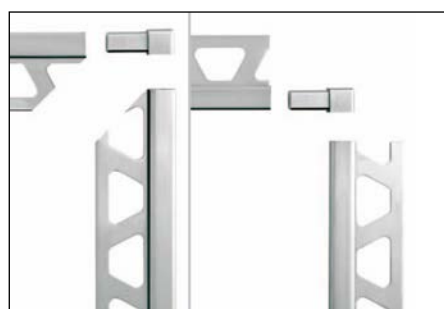
Schlüter®-QUADEC narożniki zewnętrzne i wewnętrzne
