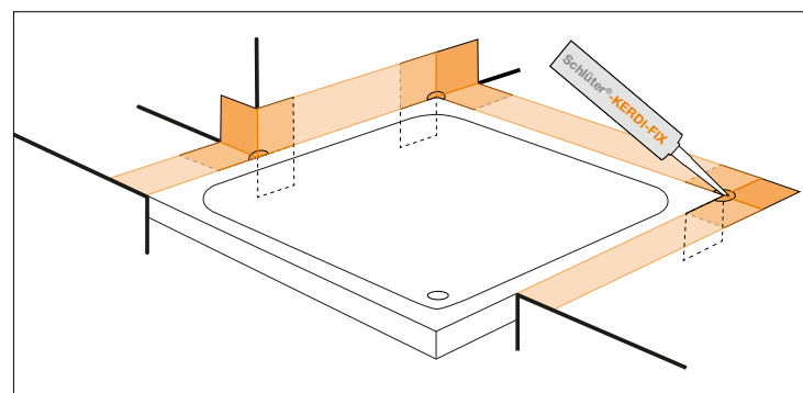
Esempi d'installazione tipo
