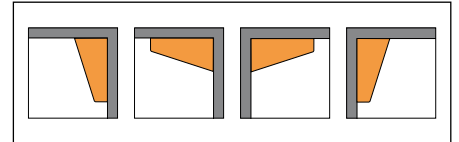
Einbaumöglichkeiten von Schlüter-SHELF-E-S3
