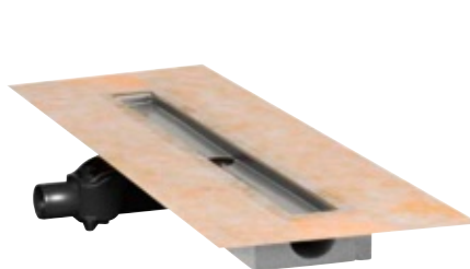
Schlüter-KERDI mandzsetta, síkban fekvő középére történő beépítéshez
