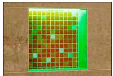
Instalación del set de hornacina Schlüter-KERDI-BOARD-NLT con iluminación acentuada
