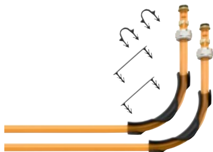
Komponenty připojovací sady pro topné potrubí Ø 16 mm
