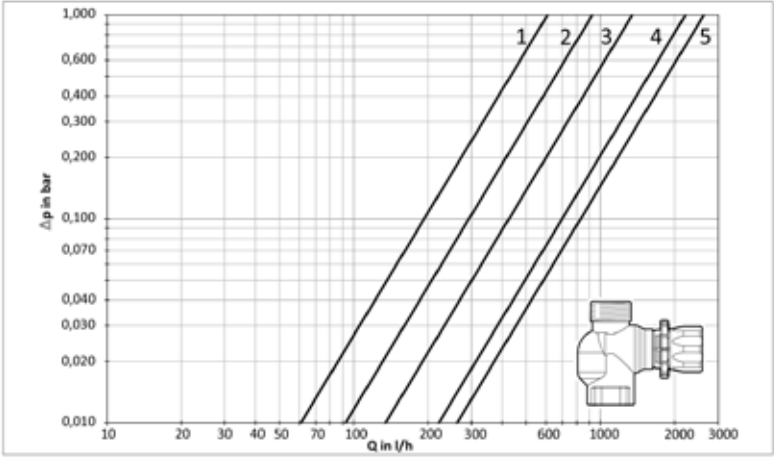
Abbildung 3: Reguliertventil
