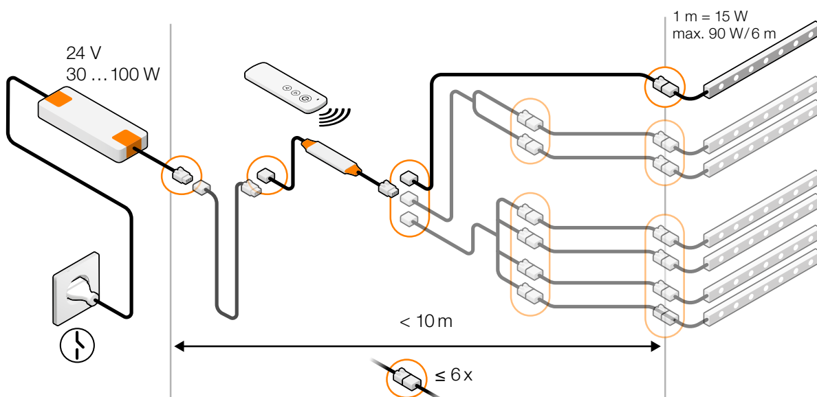
LED-Modul RGB+W
