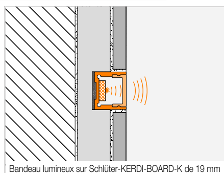
Bandeau lumineux sur Schlüter-KERDI-BOARD-K de 19 mm
