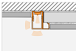
Panel ścienny na płycie Schlüter-KERDI-BOARD 19 mm
