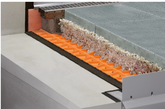
Konstrukcja okładziny na warstwie żwiru/grysu z matą drenażową Schlüter-TROBA
