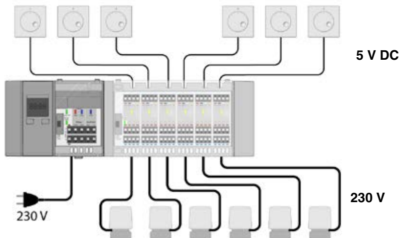
Obrázek 1: Základní modul "Control", přípojovací modul, časovač, drátová prostorová čidla a servopohony; doporučený kabel pro připojení prostorových čidel J-Y (ST) Y 2 x 2 x 0,6 mm
